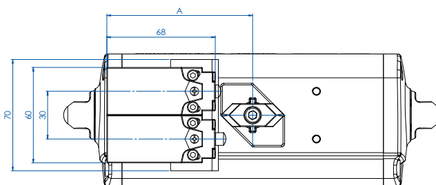
Esempio Kit con 2 Finecorsa - Example Kit with 2 Limit Switch
