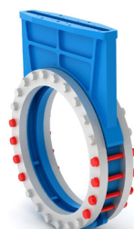
DN700÷DN800 n°24+24 fori n°32 viti + n°8 bulloni DN700÷DN800 n°24+24 holes n°32 screws + n°8 bolts
