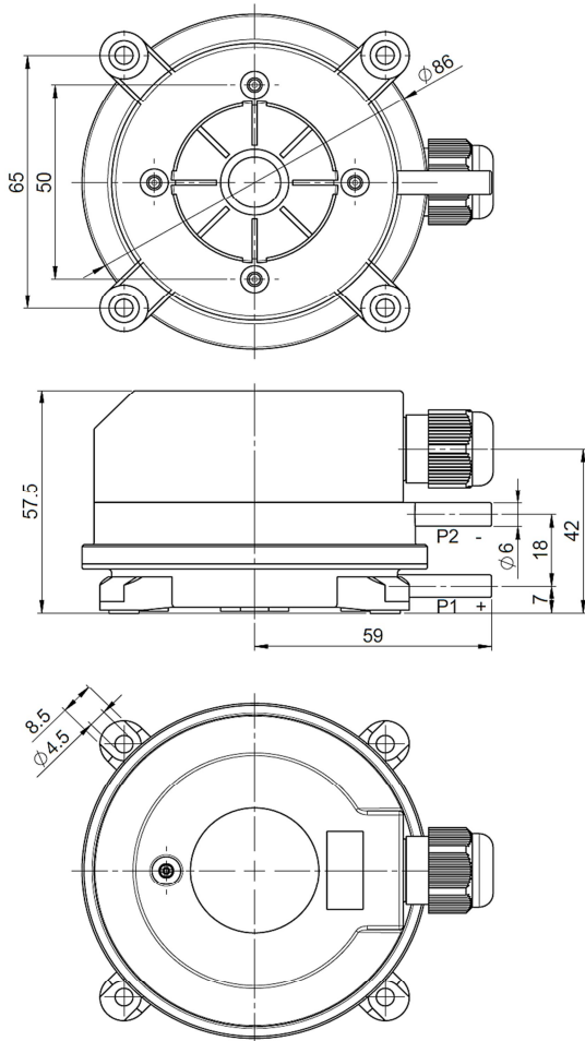
984 with cap nut conduit AF20
