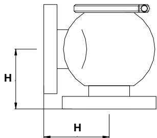
FLANGIA FLANGE
