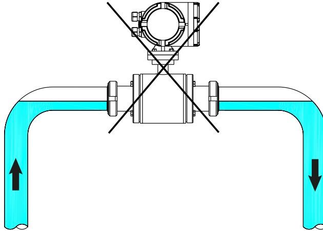
Fig.15-A Installazione nel punto superiore della tubazione
