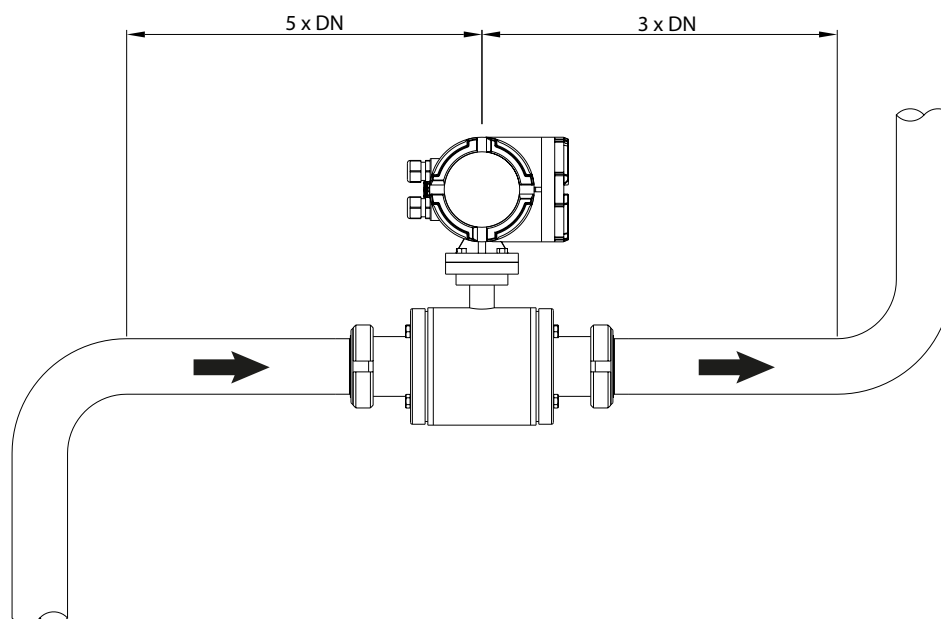
Fig.13-B. Requisiti minimi per l'installazione su tubo dritto
