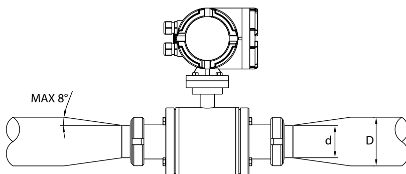
Coni di adattamento
