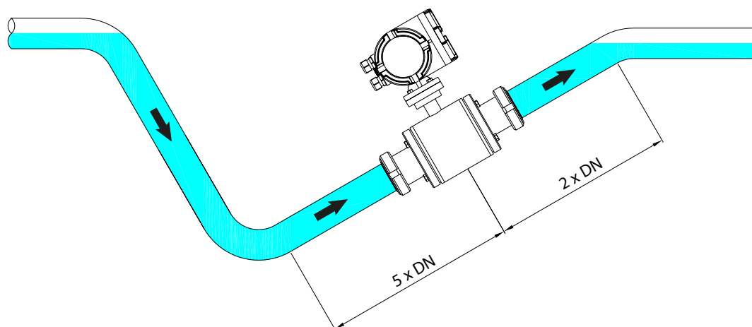
Fig.14-A Installazione in tubo parzialmente pieno
