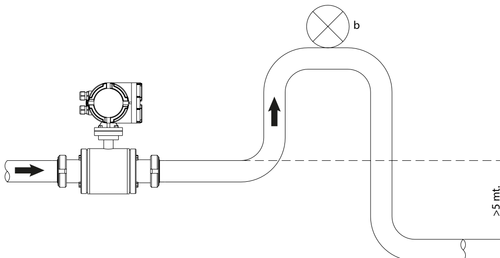
Fig.15-C Installazione in prossimità di un tratto in discesa >5m
