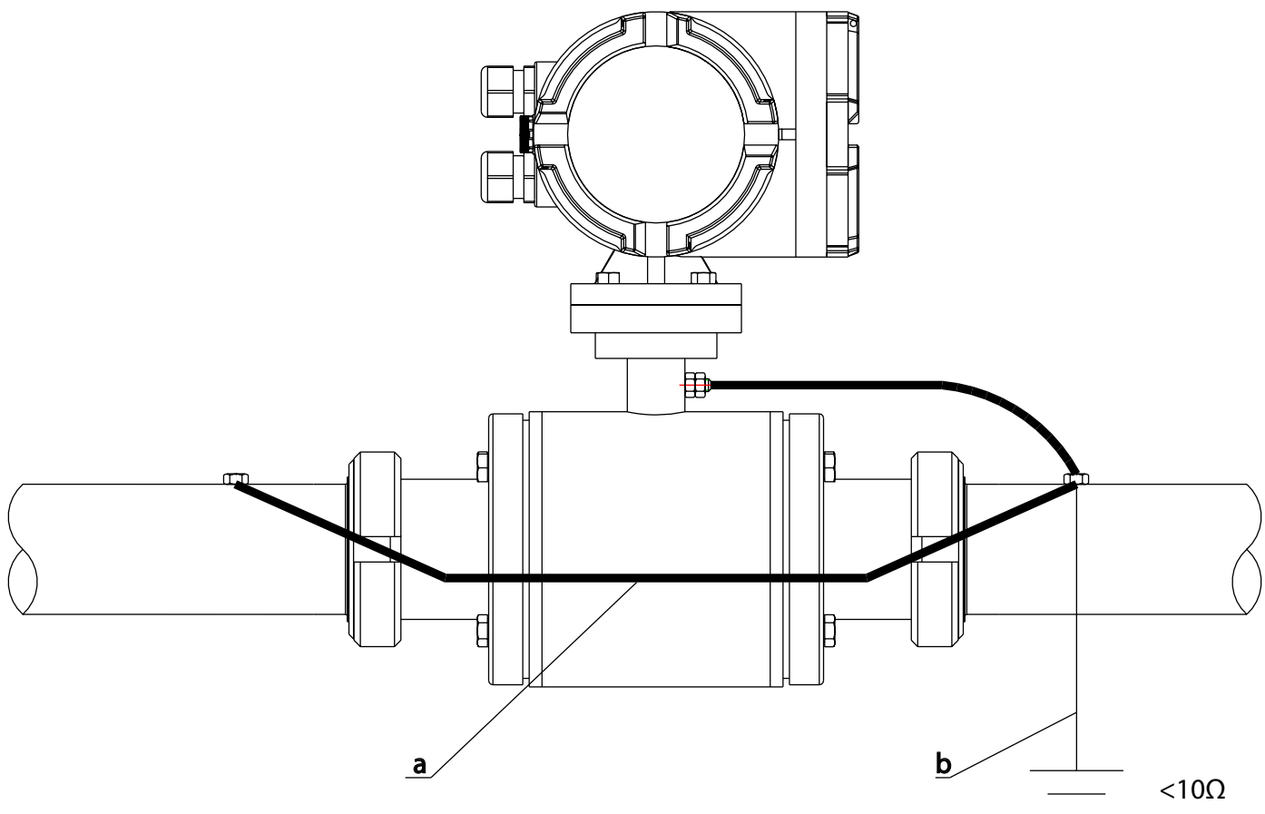
Fig.18A Schema di messa a terra
