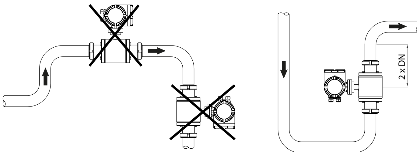
Fig.14-B Installazione in tubo senza svuotamento
