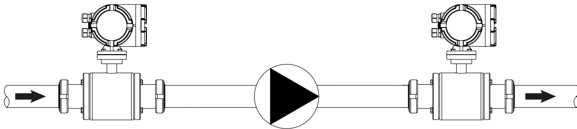
Fig.15-B Installazione in prossimità di una pompa
