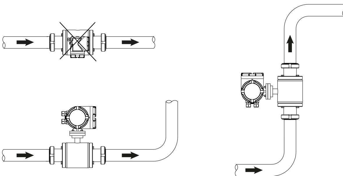
Fig.13-A. Installazione in tubo orizzontale o verticale
